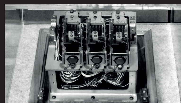
Элемент конструкции японской шифровальной машины
